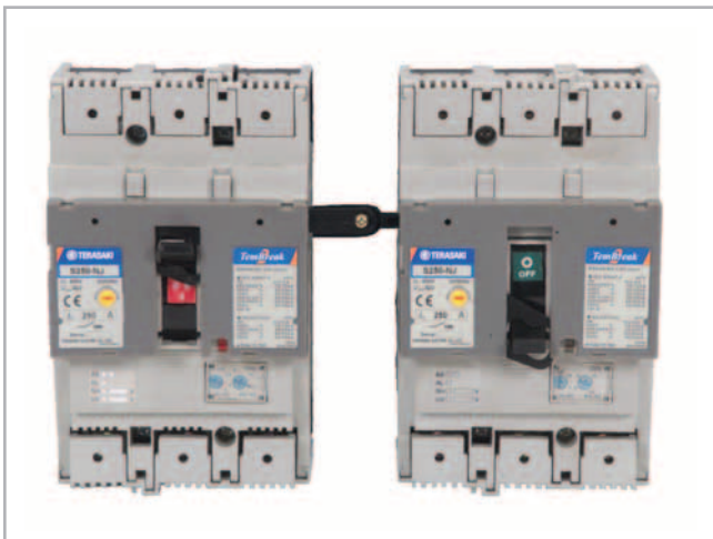
Link Interlock
